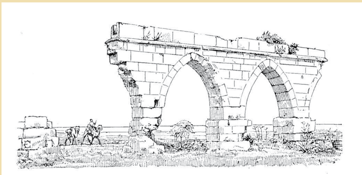
7. Τμήμα από το υδραγωγείο του Ηρακλείου, c.610, Άγιος Σέργιος Αμμοχώστου. Το υδραγωγείο προμήθευε νερό τη Σαλαμίνα – Κωνσταντία από τις πηγές του Πενταδακτύλου (σχέδιο Camille Enlart, 1896-1899). Πηγή: Enlart Camille, Gothic Art and the Renaissance in Cyprus (translated and edited by David Hunt), Trigraph, London 1987, 384.
